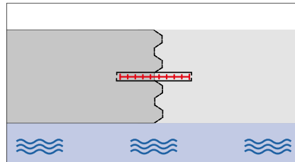
System 4 Labyrinthprinzip Verlängerung des Wasserumlauf- weg Produktgruppe: Fugenbänder
