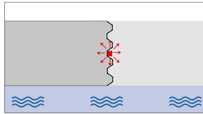
System 2 Quellprinzip durch Volumsvergrößerung Aufbau von Quelldruck Produktgruppe: quellfähige Fugenbänder
