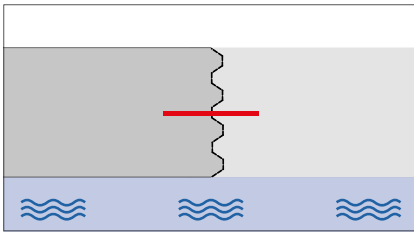
System 1 Einbettungsprinzip satte Einbettung des Profils und Haftung mit dem Beton Produktgruppe: Fugenbleche
