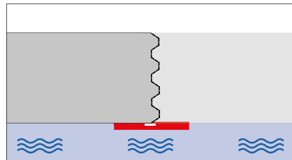
System 5 Adhäsionsprinzip Klebeverbund zwischen der Abdich- tung und dem Beton Produktgruppe: streifenförmige geklebte Abdichtung
